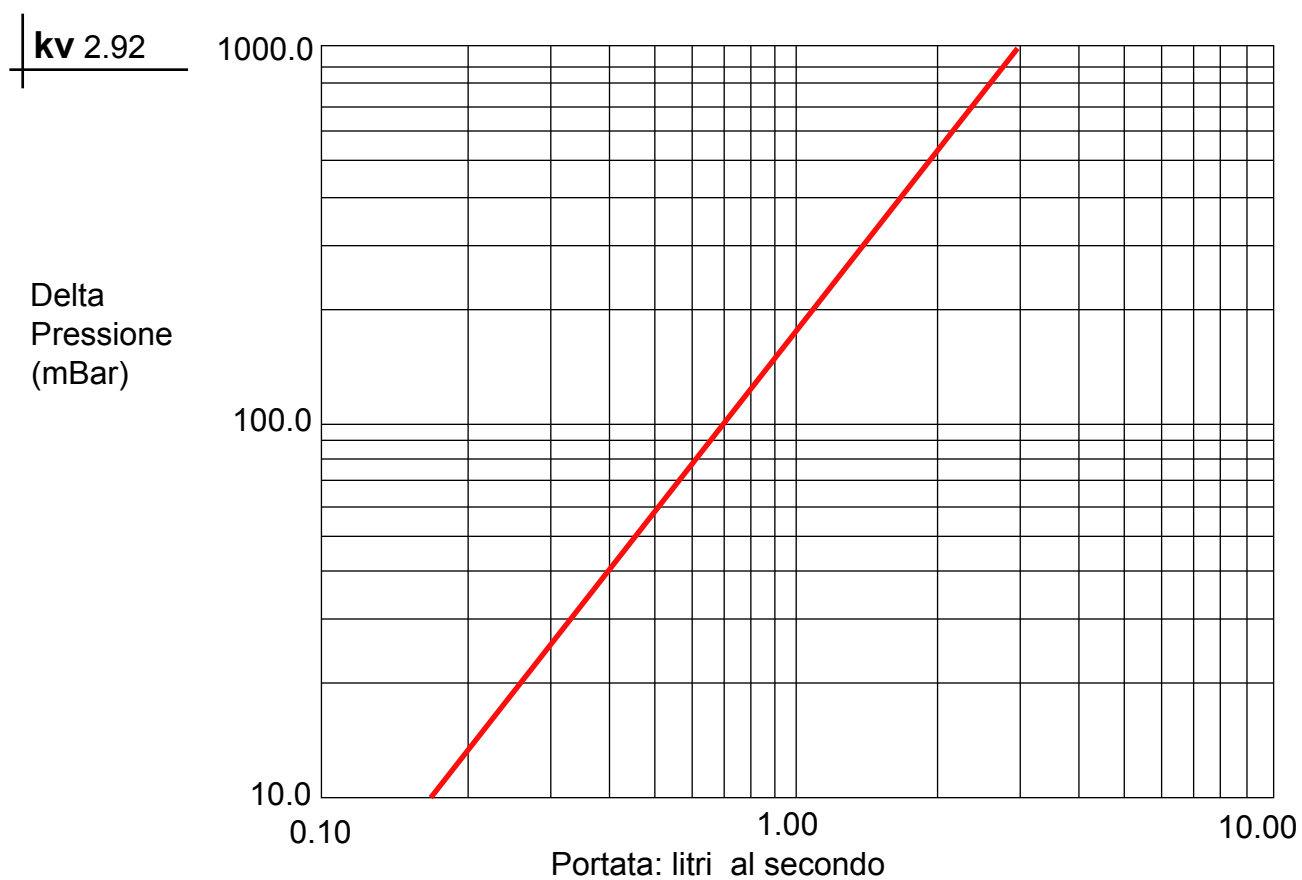
Diagramma 981559/3: determinazione della perdita di carico contro portata dell'anticalcare magnetico ELCLA2 Ø 3/4".
