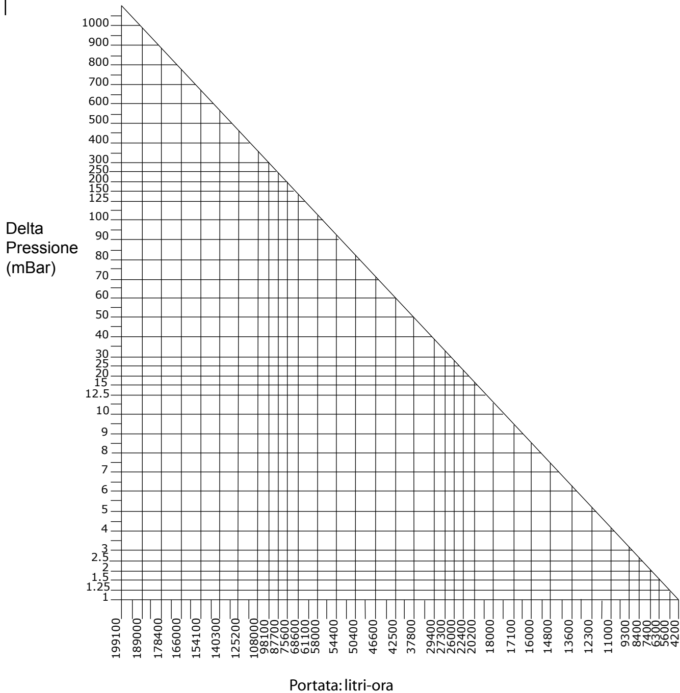
Diagramma TEST 0403101/GS/2: determinazione della perdita di carico contro portata dell'anticalcare magnetico ELCLA7 DN 80 Ø 3".
